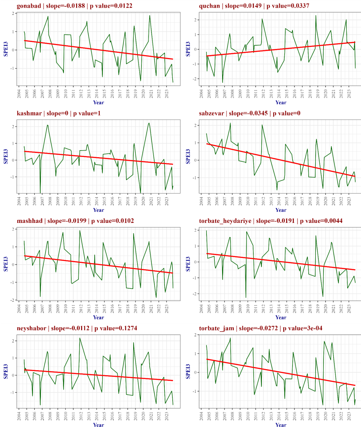
شکل ۳. نمودارهای روند خشکسالی هواشناسی در فصل پاییز بر اساس شاخص SPEI در استان خراسان رضوی طی دوره ۲۰ سال
