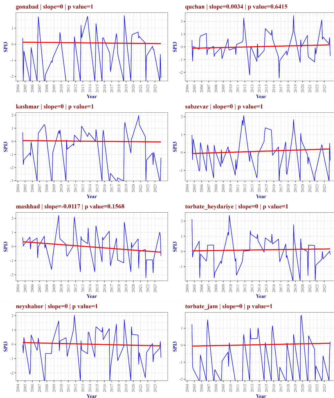
شکل ۲. نمودارهای روند خشکسالی هواشناسی در فصل پاییز برای ۲ دهه بر اساس شاخص SPI در منطقه مورد مطالعه
