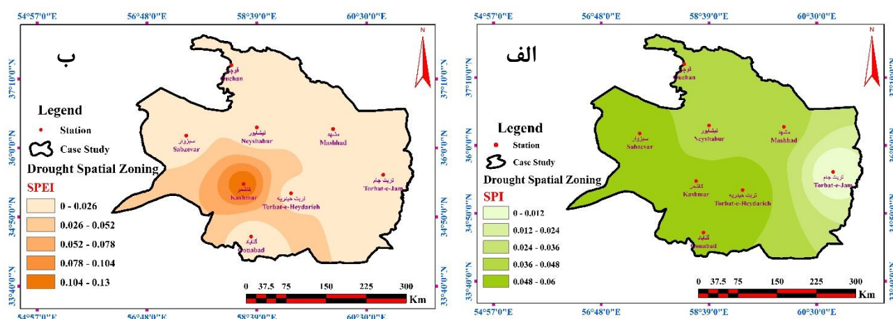
شکل ۶. نقشه‌های پهنه‌بندی منطقه مورد مطالعه در دوره ۲۰ ساله بر اساس شاخص‌های خشکسالی هواشناسی الف: SPI، ب: SPEI
