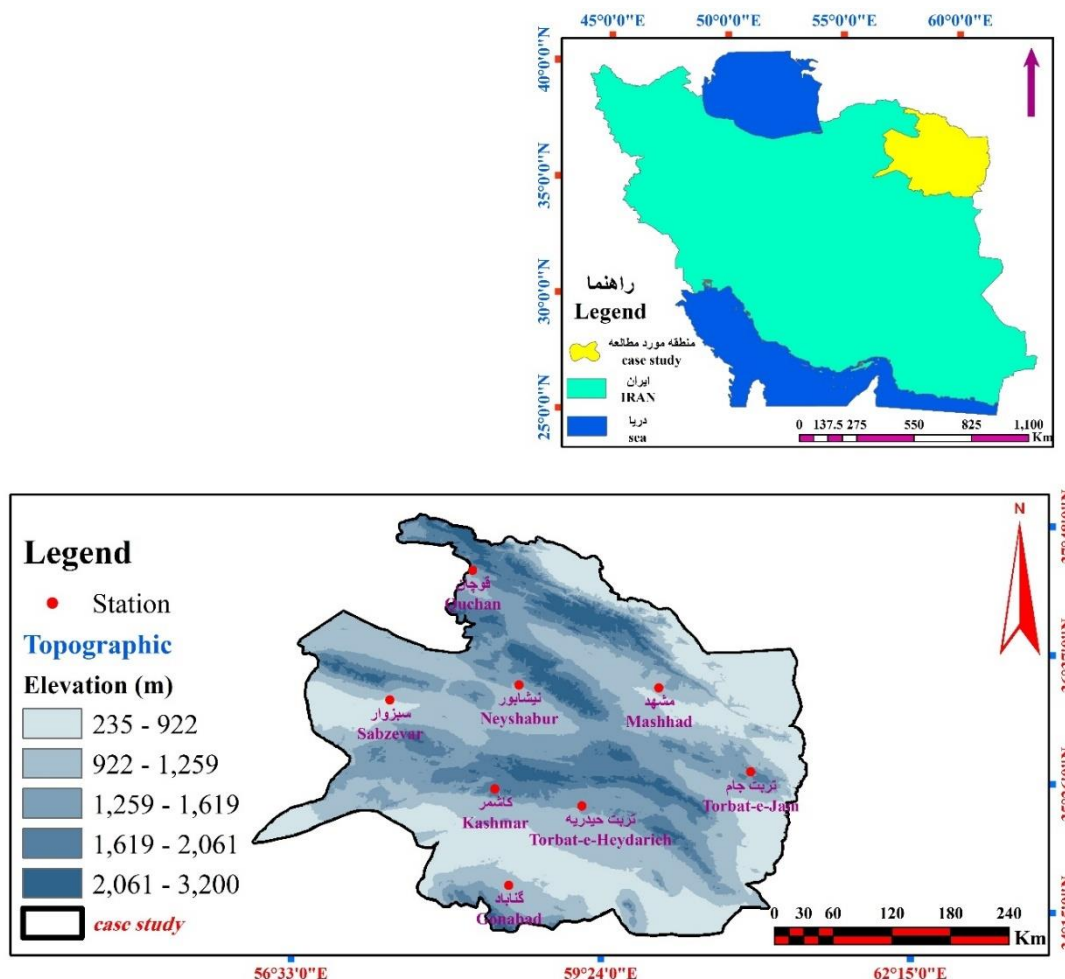
شکل ۱. موقعیت جغرافیایی منطقه مورد مطالعه، ناهمواری‌ها و ایستگاه‌های منتخب در استان خراسان رضوی Fig 1. Geographic location of the study area, topography, and selected stations in Razavi Khorasan Province
