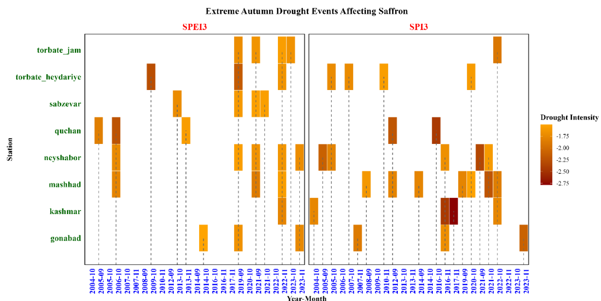
شکل ۴. نمودار هیتمپ رخدادهای حدی خشکسالی برای ۸ ایستگاه از منطقه مورد مطالعه در ۲ دهه بر اساس شاخص‌ها Fig 4. Heatmap of extreme drought events for eight stations in the study area over two decades based on the indices
