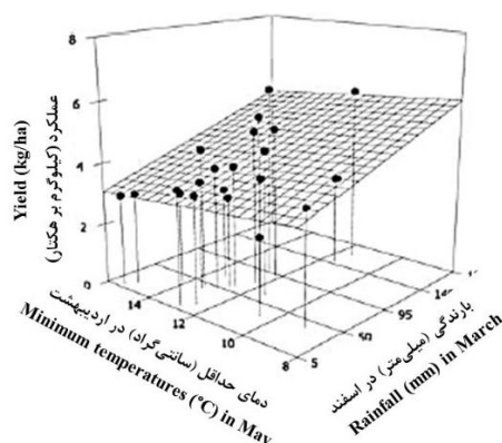
شکل ۱۰. ارتباط بین بارندگی در اسفند و دمای حداقل در اردیبهشت با عملکرد زعفران (Hosseini et al., 2008) Fig 10. Relationship between rainfall in March and minimum temperature in May with yield of saffron (Hosseini et al., 2008)
