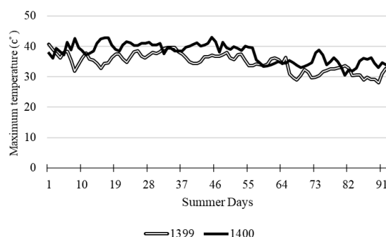
شکل ۱. حداکثر درجه حرارت روزانه تابستان سال ۱۳۹۹ و ۱۴۰۰ Fig 1. Maximum daily temperatures in the summer of 1399 and 1400
