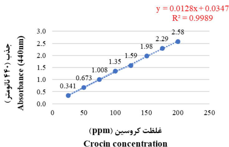
شکل ۲. منحنی استاندارد کروسین با استفاده از روش اسپکتروفتومتری
