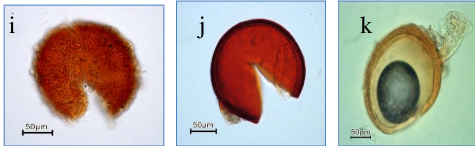
شکل ۱- مجموعه نمونه‌های قارچ میکوریزا همزیست ریشه زعفران: a: Funneliformis caledonium , b,c,d: Claroideoglosum etunicatum , e: Glomus microaggregatum , f: Funneliformis mosseae , g: Glomus aggregatum , h: Entrophospora infrequens , i: Glomus tortusum , j: Septoglosum constrictum , k: Glomus fasciculatum .
